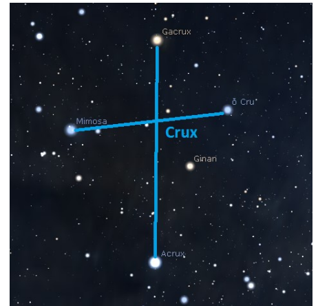
Созвездие Креста
