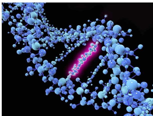
Мутация ДНК
