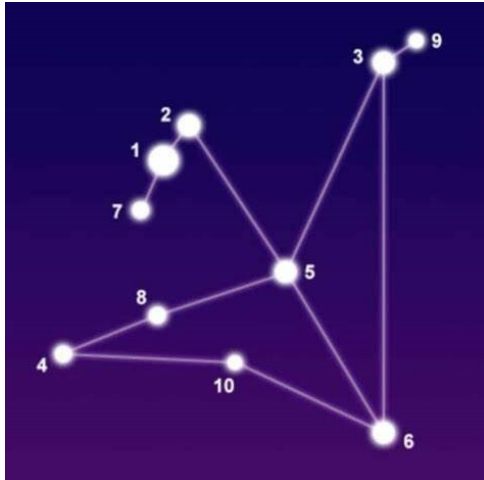
Созвездие Орла
